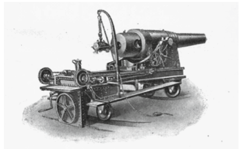
24-cm oder 96-Pfünder Krupp Ringkanone – max. Schussweite 8.000 m
